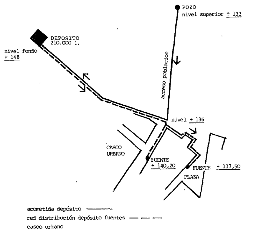
ESQUEMA DE ACOMETIDA DESDE POZO A DEPOSITO EXISTENTE EN LES VENTALLAS (ULLDECONA) Y DISTRIBUCIÓN DESDE ESTE HASTA DOS FUENTES PUBLICAS
